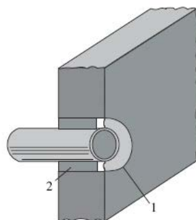
Abbildung 3: Rohrdurchführung.
