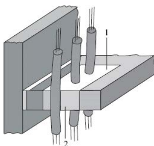
Abbildung 3: Rohrdurchführung.
